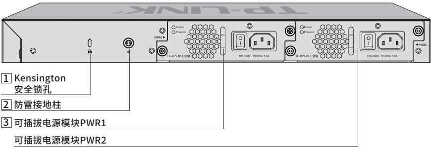
图1-2 TL-SG5428工业级后面板示意图
