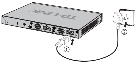
图3-4 电源线连接示意图
