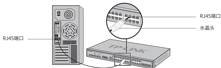
图3-1 RJ45端口连接示意图
