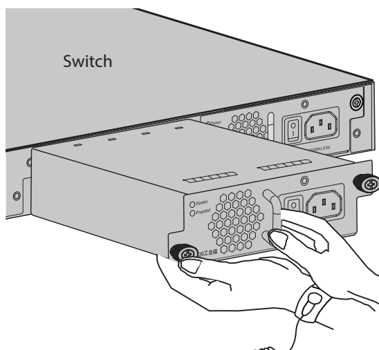
图3-5 安装电源模块示意图
