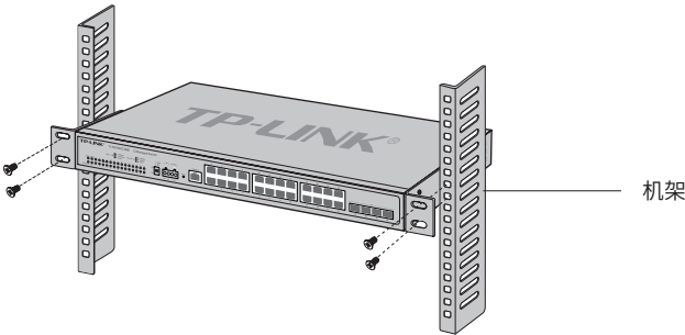
图2-3 机架安装示意图
